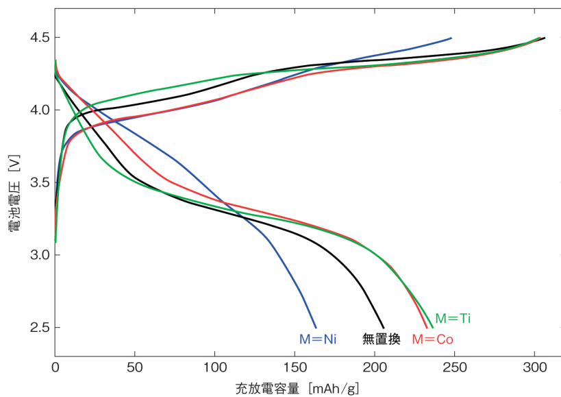
[1.1.1.2] 図2 新規ベースメタル正極活物質 (\text{Li}_{1+x}(\text{Fe}_{0.4}\text{Mn}_{0.4}\text{M}_{0.2})_{1-x}\text{O}_2) 、 0 < x < 1/3 、 \text{M}=\text{Ti} 、 \text{Co} 、 \text{Ni} および \text{Li}_{1+x}(\text{Fe}_{0.5}\text{Mn}_{0.5})_{1-x}\text{O}_2 の 60^\circ\text{C} における充放電初期特性 (p.35)
